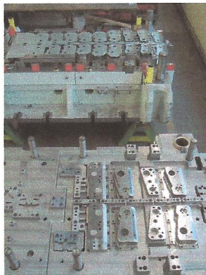
Ober- und Unterteil des Folgeverbundwerkzeugs.
