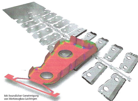
Streifenbild des Schliessblechs und in AutoForm simuliertes Bauteil.
