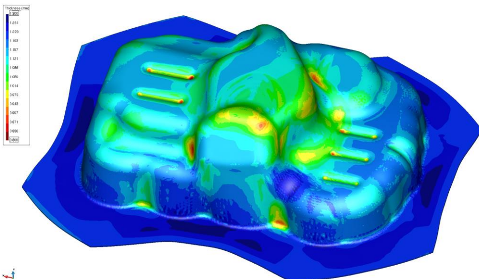
Vorhersage der Ausdünnung durch eine Simulation mit Stampack. (Alle Bilder: Stampack GmbH)
